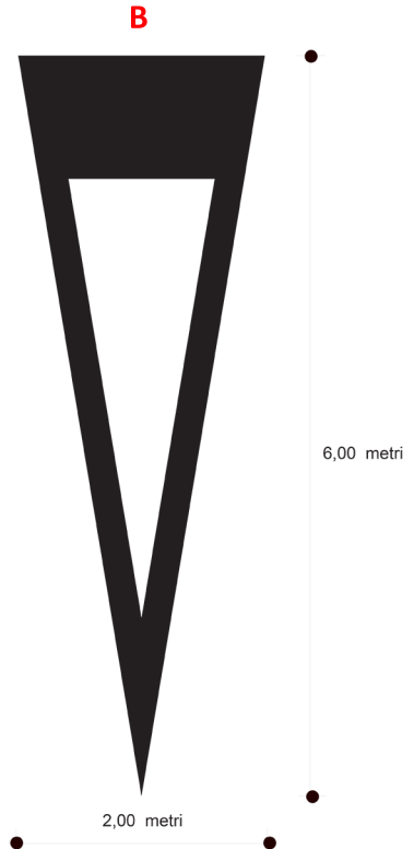
Figura II 442/a Reg. - C.d.S. - Art. 148 SIMBOLO SULLA PAVIMENTAZIONE Triangolo elongato complementare del segnale verticale DARE LA PRECEDENZA SU STRADE DI TIPO A-B-C-D
