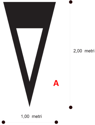
Figura II 442/a RIDOTTO Reg. - C.d.S. - Art. 148 SIMBOLO SULLA PAVIMENTAZIONE Triangolo elongato complementare del segnale verticale DARE LA PRECEDENZA SU STRADE DI TIPO E-F
